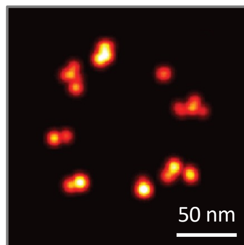
MINFLUX
