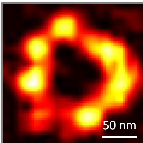
STED
